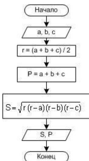
Рисунок 2 - Алгоритм примера 1
